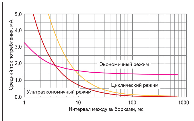
Рис. 13. Зависимость тока потребления AS5030 от частоты выборки с учетом выбранного режима работы
