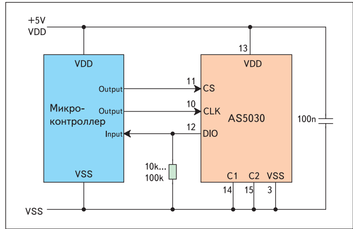
Рис. 5. Схема 3-проводного подключения в режиме «только чтение»
