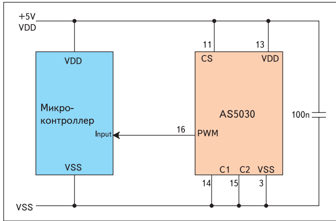
Рис. 7. Схема подключения AS5030 с использованием ШИМ-выхода
