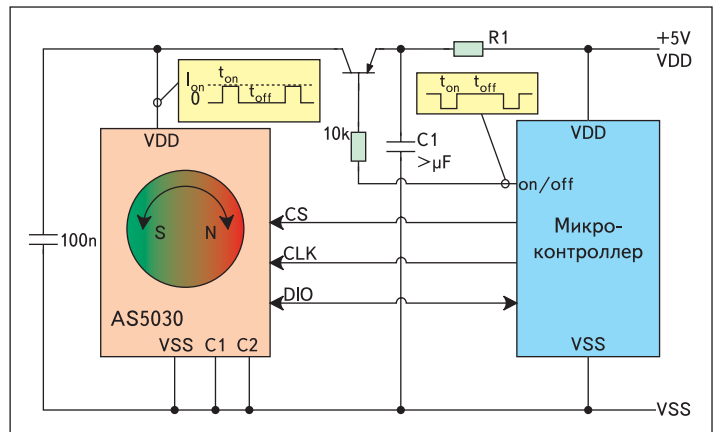
Рис. 12. Подключение AS5030 при циклическом режиме работы
