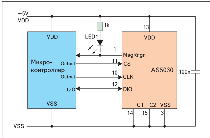
Рис. 3. Типовая схема 3-проводного подключения через SSI интерфейс
