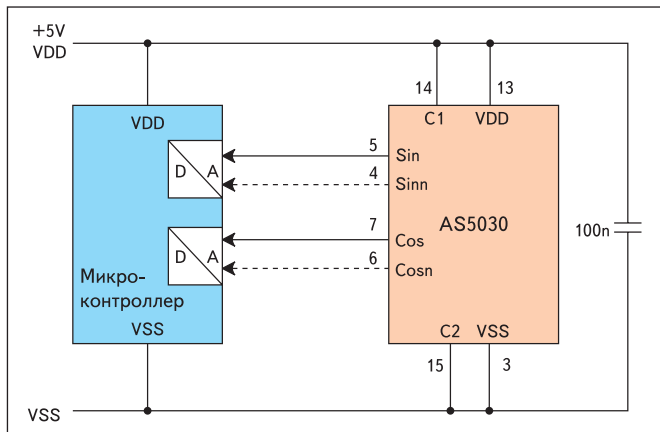
Рис. 11. Подключение AS5030 к внешнему АЦП
