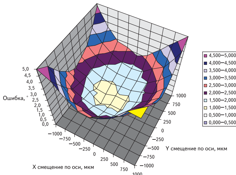
Рис. 14. Зависимость величин ошибок, возникающих при отклонении центра магнита от диагонального центра микросхемы
