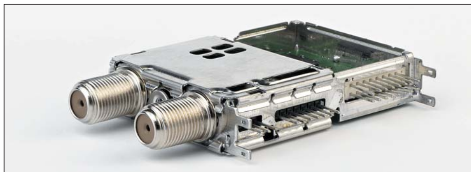
Рисунок. Тюнер DVB-T NIM Sharp VA 1K5ED6255
