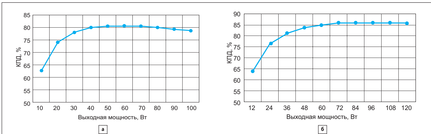
Рис. 3. Зависимость КПД от выходной мощности при T_A = 25^\circ\text{C} и входном напряжении 100 В модуля: а) HDCC/100W-5-100U/SP; б) HDCC/100W-28-120U/SP
