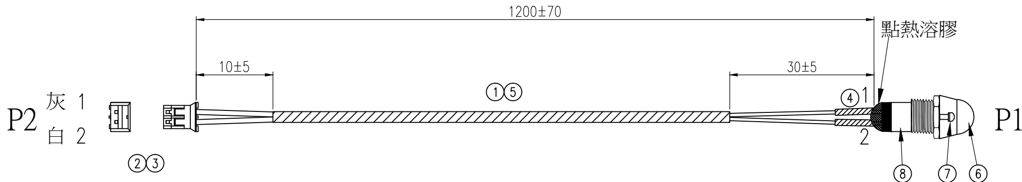
WIRING TABLE
